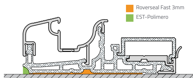
Esempio di applicazione di nastro Roverseal Fast 3 da 50mm su soglia ST570 . Scala 1:1.
