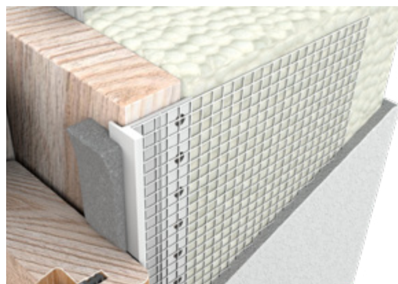
Profilo di finitura 6 mm
